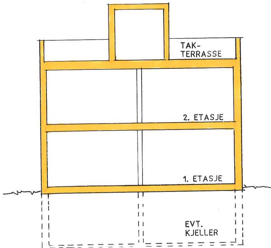
SNITT
