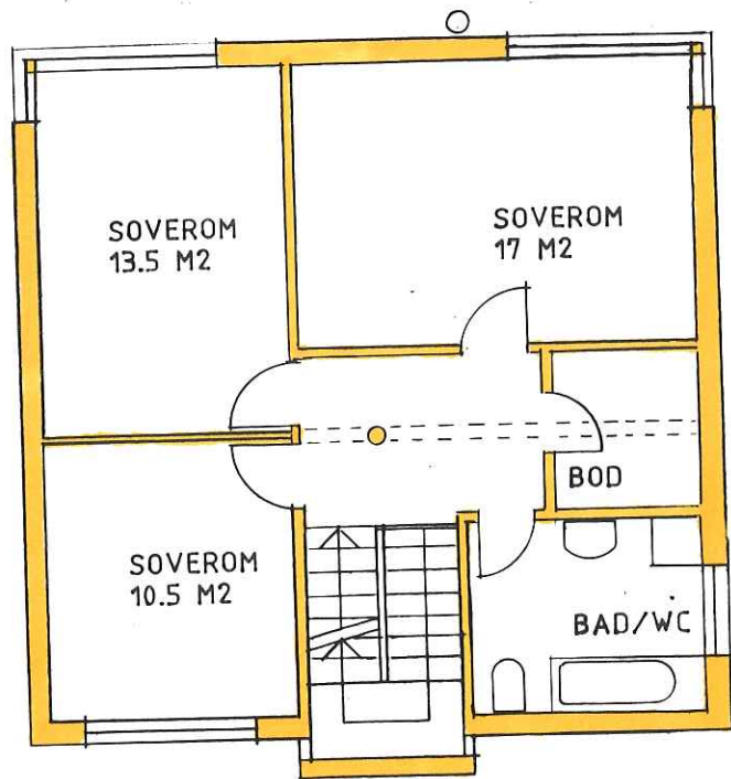
PLAN 2. ETASJE
