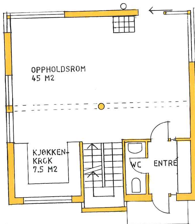
PLAN 1. ETASJE
